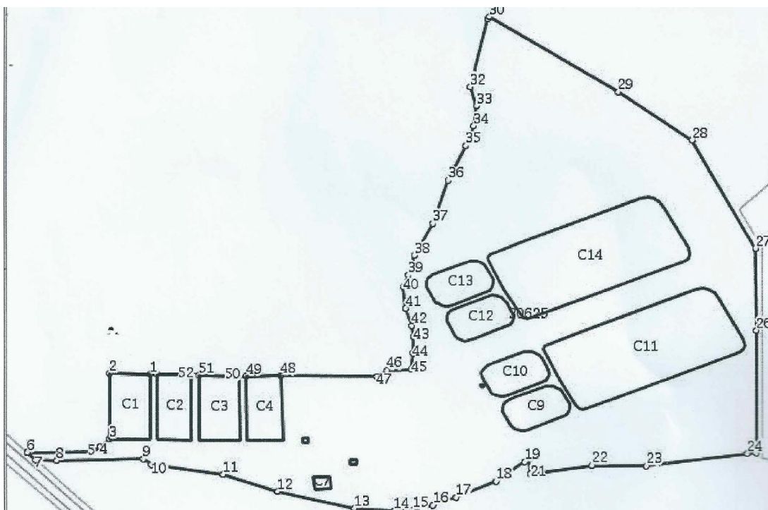
Fig. 2 – amplasament instalatie biogaz
