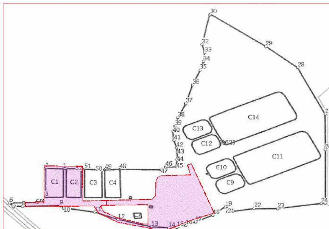
Fig. 2 – amplasament instalatie cogenerare
