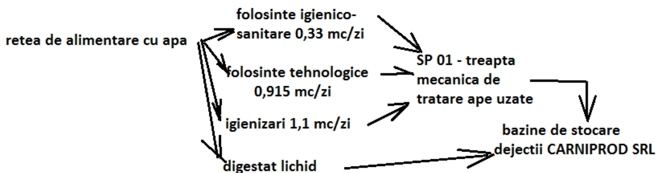
Fig. Procesul apei menajere si a apei pentru spalare
